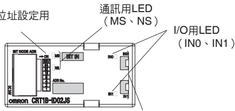
本體正面 I/O接頭配置顯示
