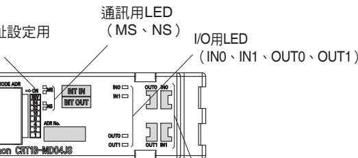
本體正面 I/O接頭配置顯示
