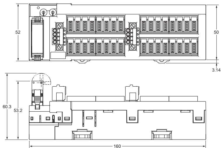
安裝開放型接頭 (DCN4-TB4型) 時
