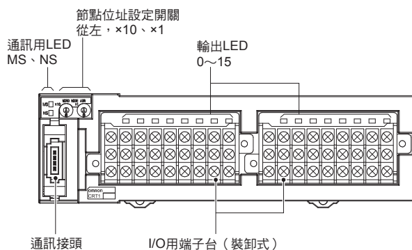
CRT1-OD16TA (-1) 型、CRT1-OD16TAH (-1) 型
