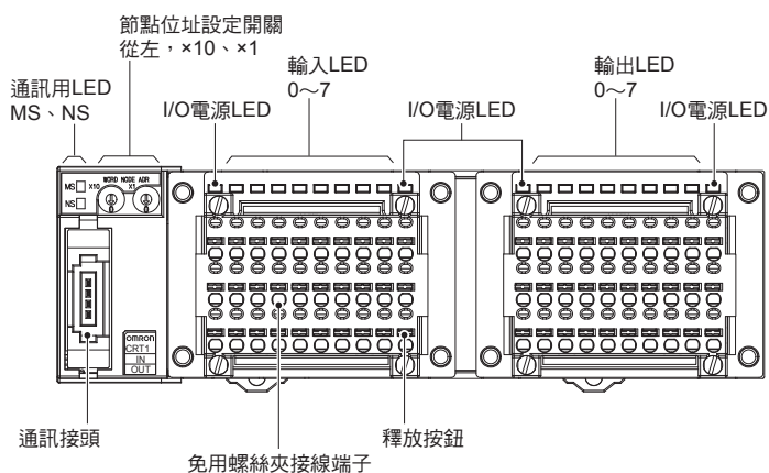
CRT1-MD16SL型、CRT1-MD16SL-1型
