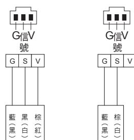
NPN輸出3線式感測器 (光電開關、近接開關) 2線式感測器 (限動開關等)
