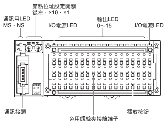
CRT1-OD16SL型、CRT1-OD16SL-1型
