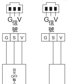
光電開關、投光機等 電磁閥等 閥件
