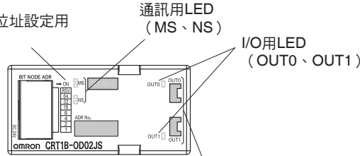
本體正面 I/O接頭配置顯示
