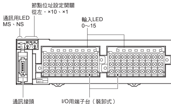
CRT1-ID16TA (-1) 型、CRT1-ID16TAH (-1) 型
