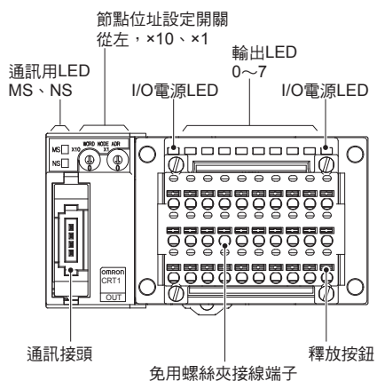
CRT1-OD08SL型、CRT1-OD08SL-1型
