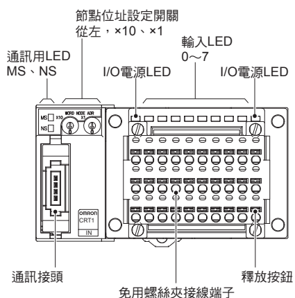
CRT1-ID08SL型、CRT1-ID08SL-1型
