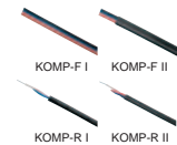
CompoNet扁平纜線I、II CompoNet圓形纜線I、II ①CompoNet扁平纜線I KOMP-F I : 21AWGx2、19AWGx2 ②CompoNet扁平纜線II KOMP-F II : 21AWGx2、19AWGx2 ③CompoNet圓形纜線I KOMP-R I : 19AWGx2 ④CompoNet圓形纜線II KOMP-R II : 19AWGx4
