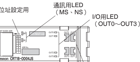
本體正面 I/O接頭配置顯示
