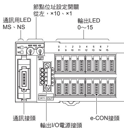
CRT1-OD16S (-1) 型、CRT1-OD16SH (-1) 型
