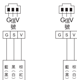
PNP輸出3線式感測器 (光電開關、近接開關) 2線式感測器 (限動開關等)
