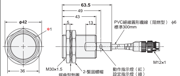
E2EF-X12D1-M1TGJ型 E2EF-QX12D1-M1TGJ型
