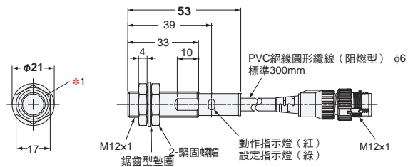
E2EF-X3D1-M1TGJ型 E2EF-QX3D1-M1TGJ型
