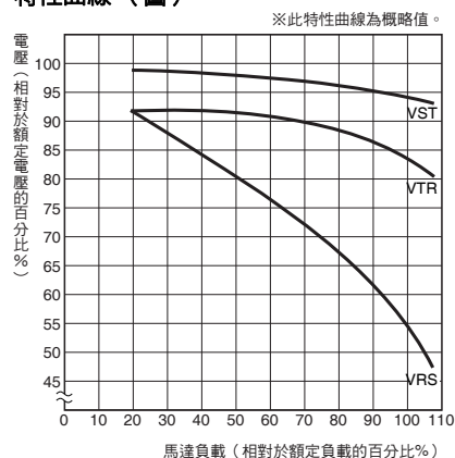
特性曲線 (圖)
