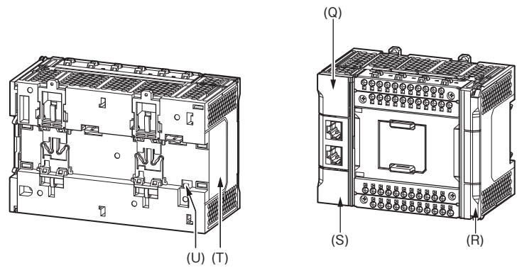
NX1P2-9024□□□型
