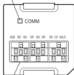
RS232C端子台
