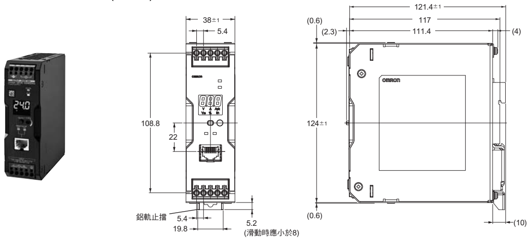
上圖所示為S8VK-X24024A-EIP型。
