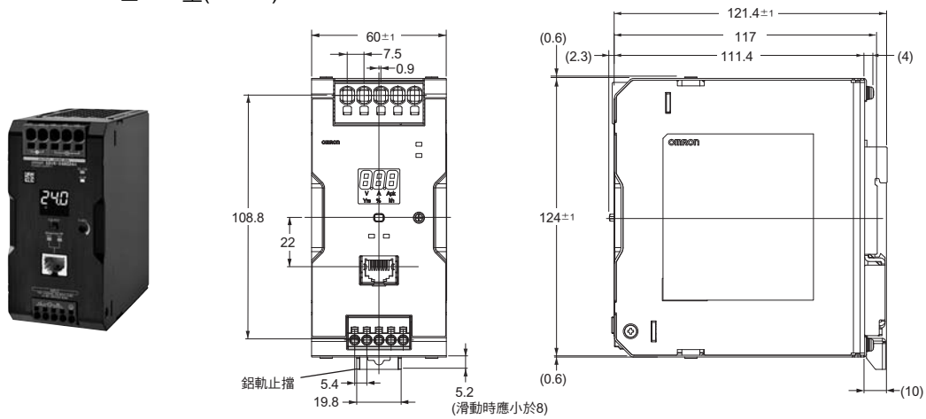
上圖所示為S8VK-X48024A-EIP型。
