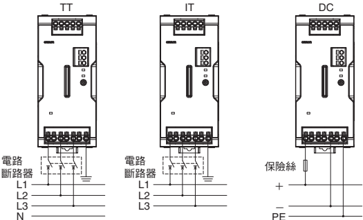
輸入的配線（TT、IT、DC）
