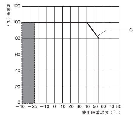
240W/480W/960W &lt;左右間隔不到15mm&gt;
